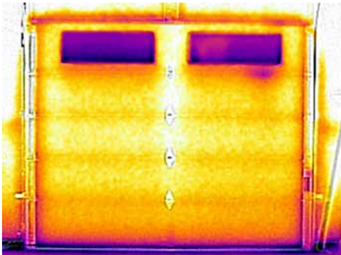
THERMOGUARD™ DOOR
